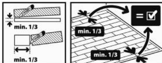
Pokládka podélně
